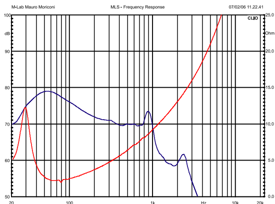
Risposta in frequenza Curva di impedenza
